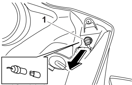
1. Standlichtlampe
