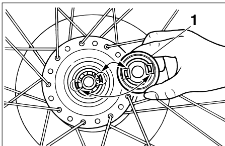
1. Módulo de engrenagens do velocímetro
