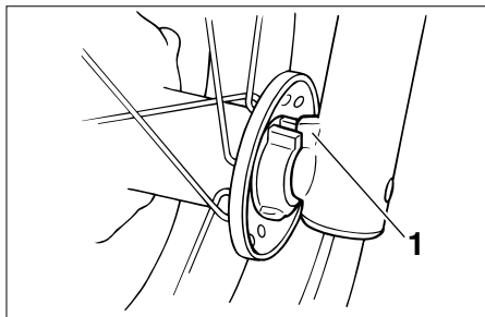
1. Retentor do módulo de engrenagens do velocímetro
