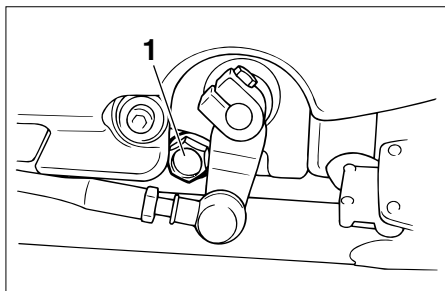
1. Cavilha de drenagem de óleo do motor
