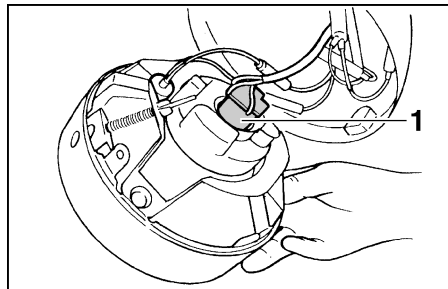
1. Stekker koplampbedrading
