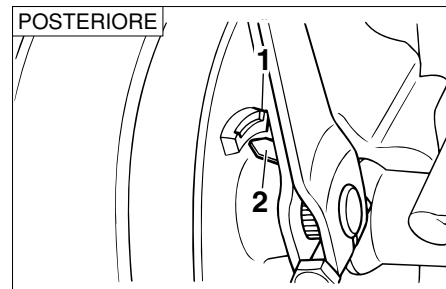
1. Limite d'usura 2. Indicatore di usura
