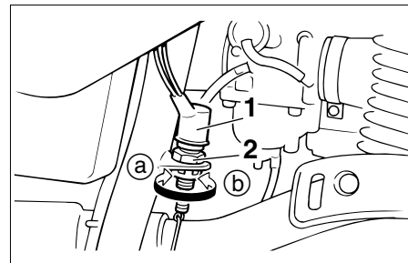
1. Interruttore della luce dello stop 2. Dado di registro
